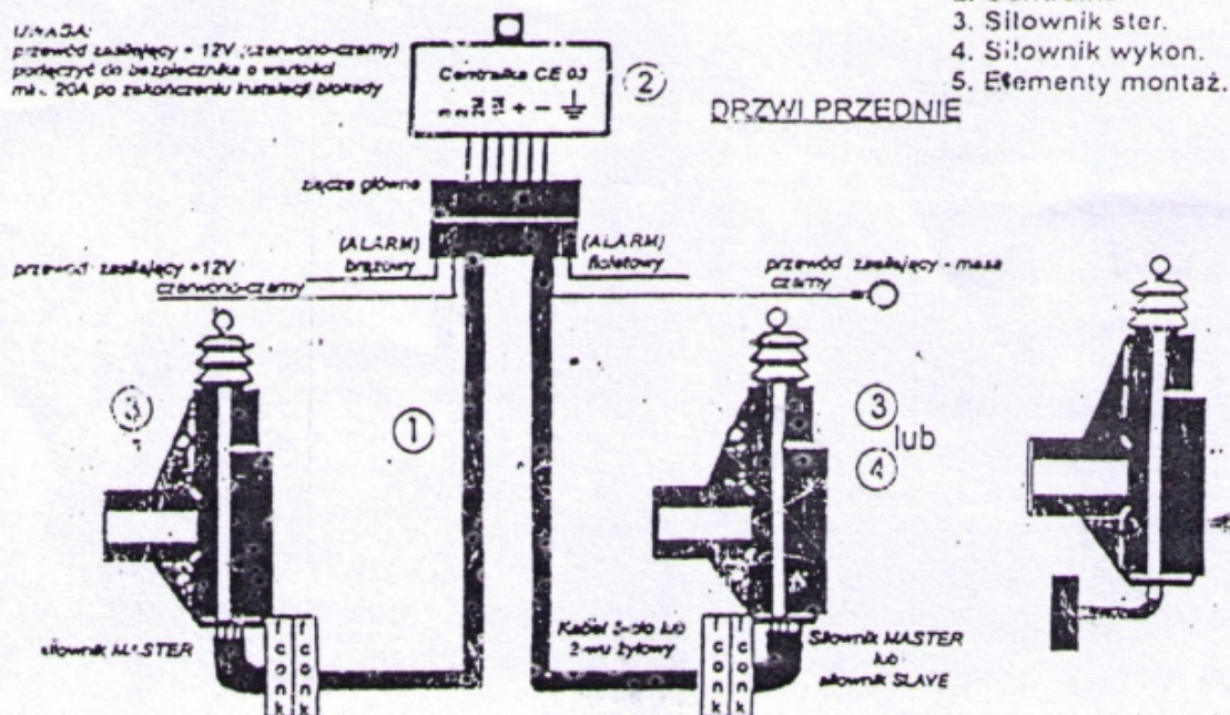
SCHEMAT IDEOWY CENTRALNEJ BLOKADY ZAMKÓW
